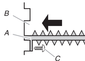
A. Cortina lateral contra la ranura de la ventana B. Ranura de la ventana C. Tornillo de cabeza redonda #8 x 3/4"
